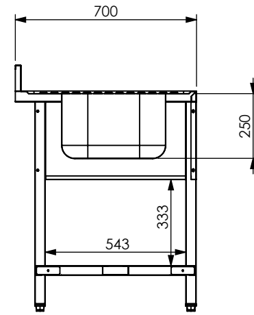
KESIT A-A
